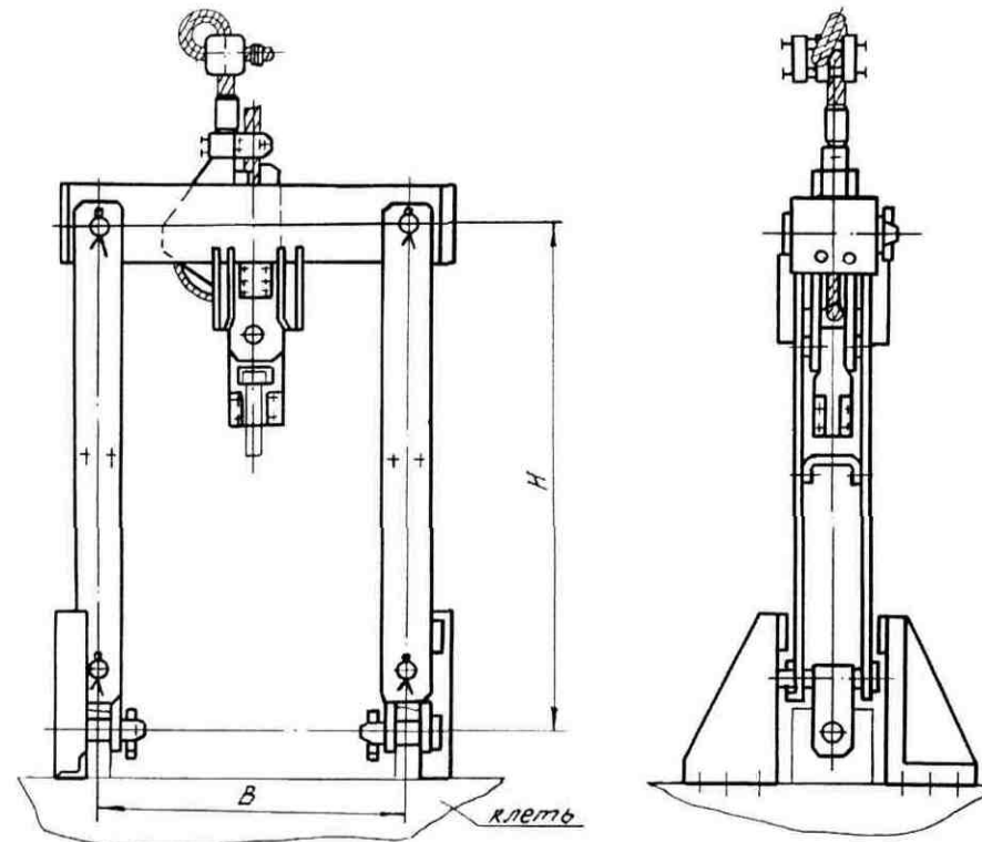
Основные параметры и размеры подвесных устройств УП для шахтных клетей
