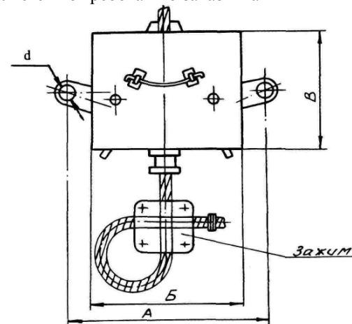
Параметры коушей
